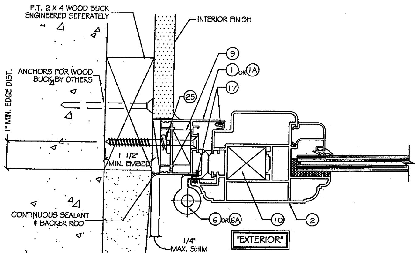
1 JAMB DETAIL (CONC. SUBSTRATE) 4 SCALE: 1/4" = 1'-0"
